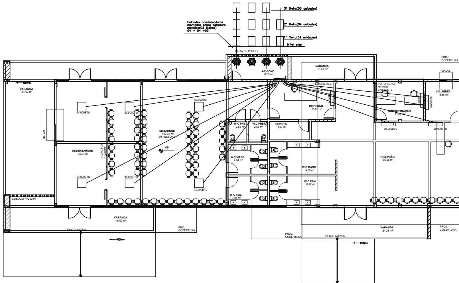
PLANTA BAIXA PAVIMENTO TERREO - AR-CONDICIONADOS ESC. 1/75
