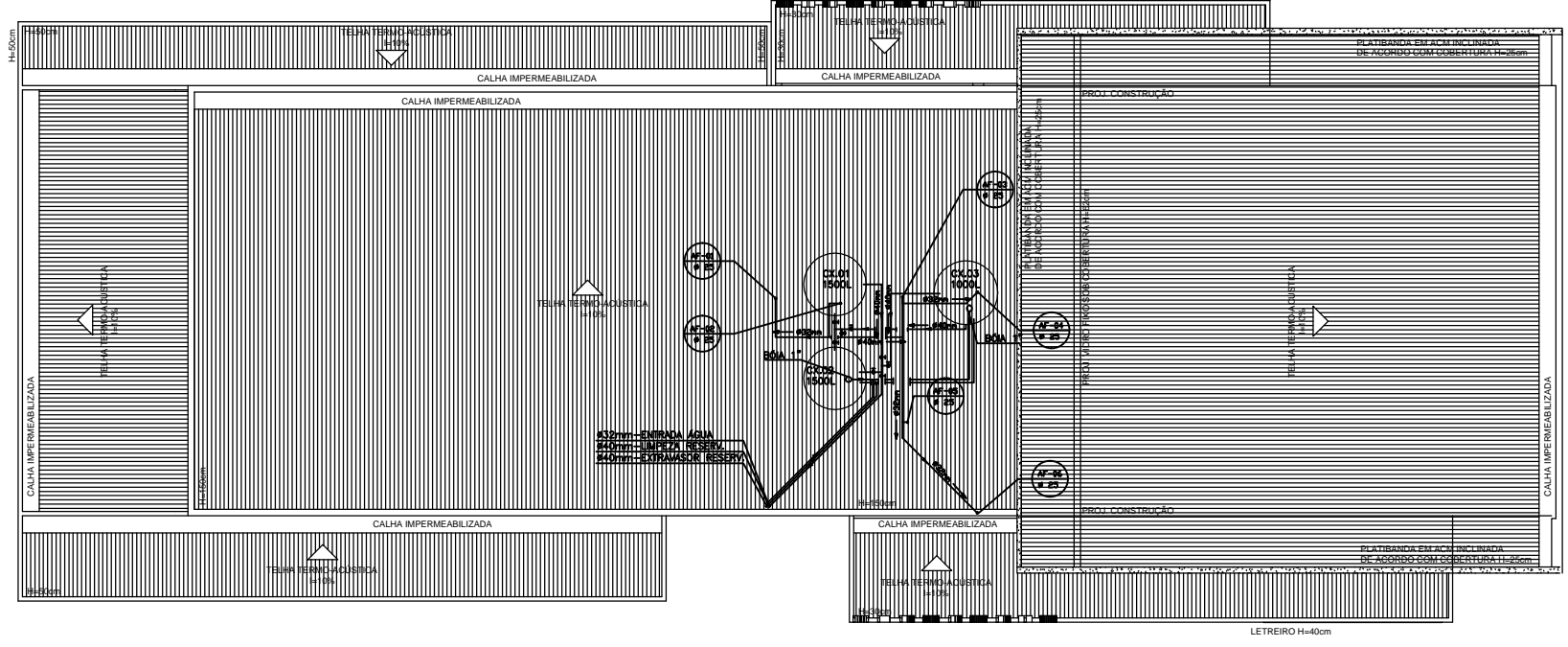
PLANTA BAIXA COBERTURA ESCALA: 1/75
