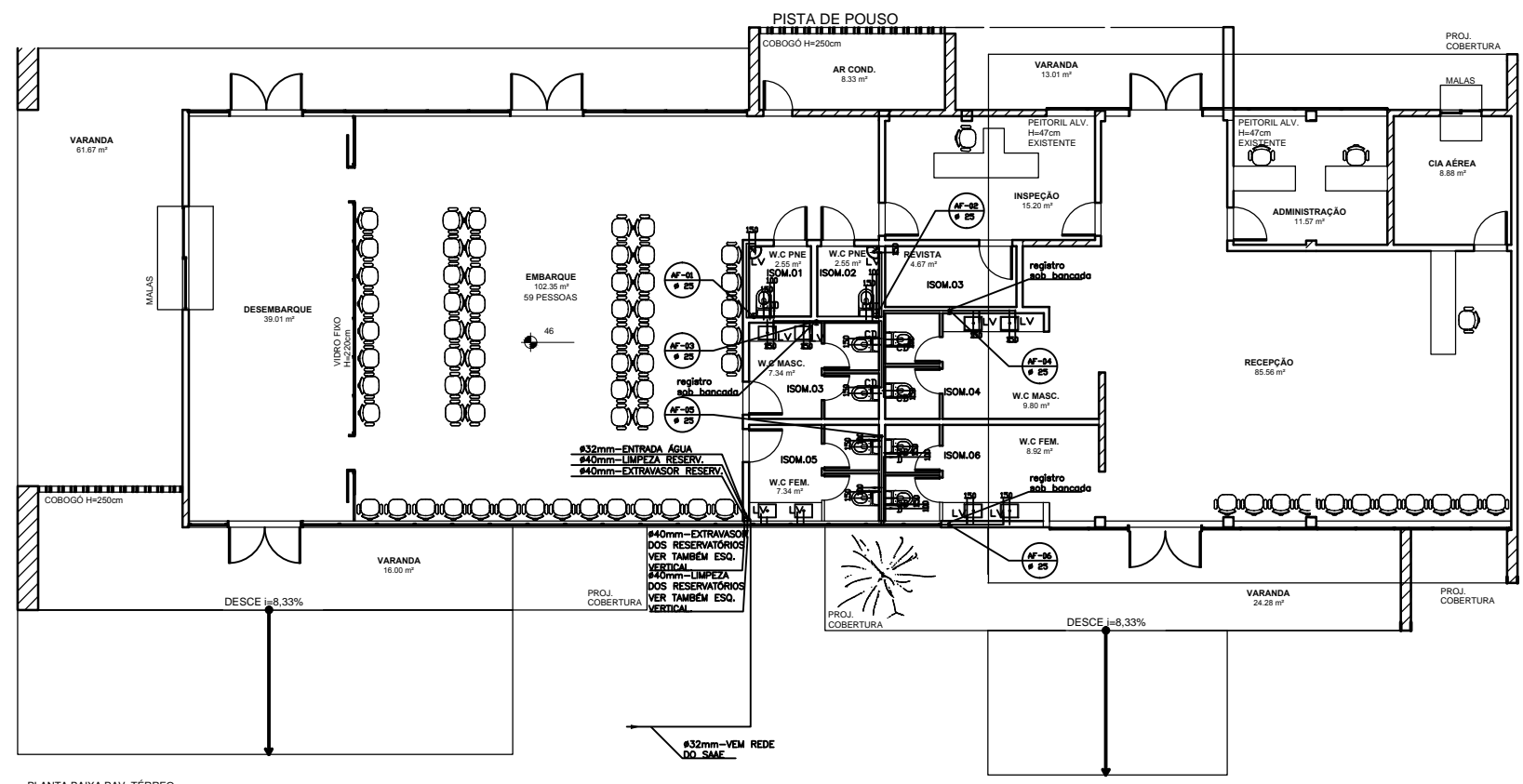
PLANTA BAIXA PAV. TÉRREO ESCALA: 1/75
